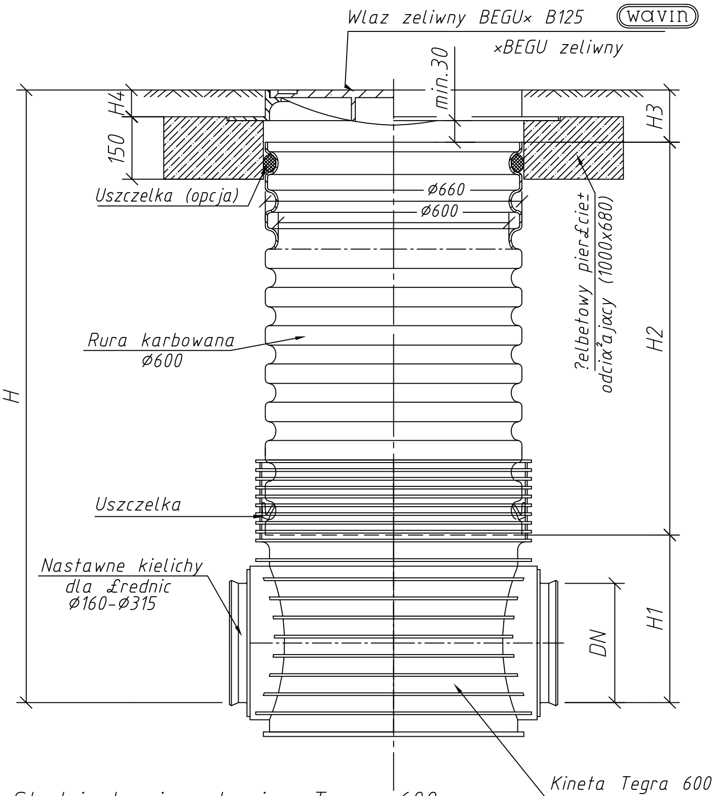
Studzienka inspekcyjna Tegra 600 z żelbetowym pierścieniem odciażającym oraz włazem klasy B125
